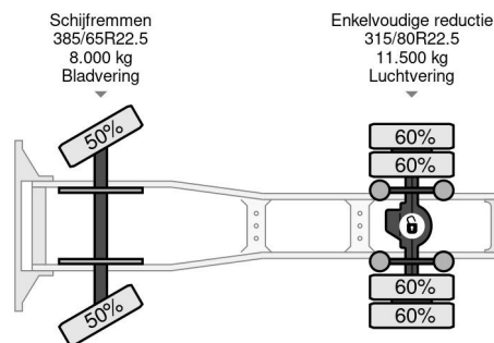
Volvo FH 460 4X2 EURO 6 STANDKLIMA
