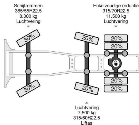
Volvo FH 500 6X2 EURO 5
