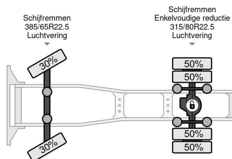
Volvo FH 500 4X2 I SHIFT EURO 6
