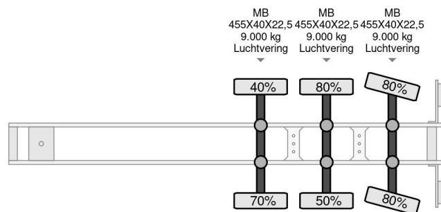
TRACON TRAILERS LZV MET SCHOTEL LIFT EN STUURAS
