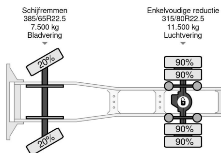
Scania R490 4X2 EURO 6 + ADR RETARDER
