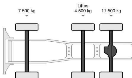
Volvo FH 460 6X2 EURO 6 ADR i-Shift i-ParkCool
