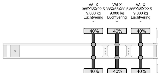
Knapen Trailers K100, 1E + 3E LIFT AXLE, REMOTE CONT...
