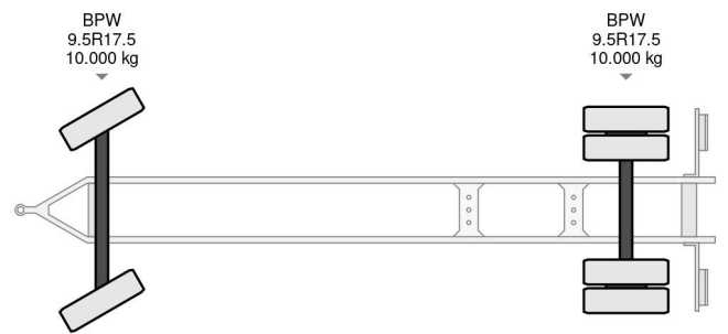
Burg BPA 10-10 ARXXX 2X BPW AXLE // TÜV TILL 01-2025
