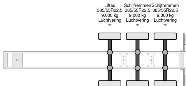
Hertoghs O3 / BOX TRAILER 3X SAF AXLE
