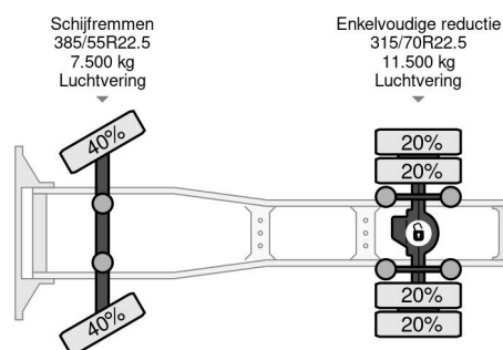
Scania R450 4X2 EURO 6 SKIRTS STANDKLIMA
