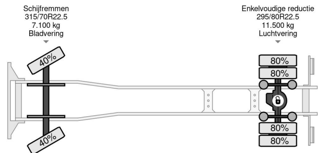
Mercedes-Benz Atego 1823 4X2 - PUTZMEISTER M24-20 R...
