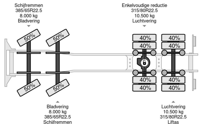
MAN TGA 35.440 8X2 - EURO 4 + HMF 2620K-RC 2018! + ...
