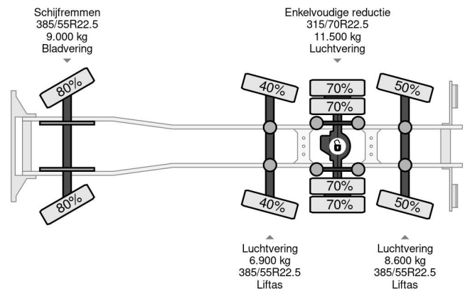
Scania P360 8X2 - HIAB 211BW-3 + FAUN VARIOPRESS - ...
