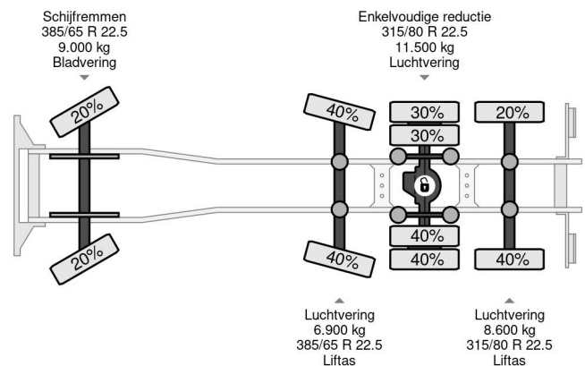
Scania R490 8X2 EURO 6 RETARDER
