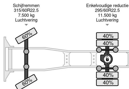
Mercedes-Benz Actros 1842 4X2 - EURO 6 + HEFSCHOTEL ... Referenznummer: MB118370
