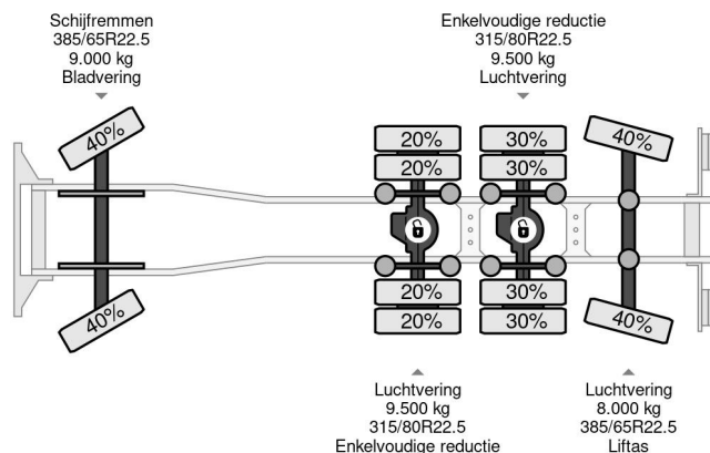
MAN TGX 35.500 8X4 VAKO BANDLOSSER
