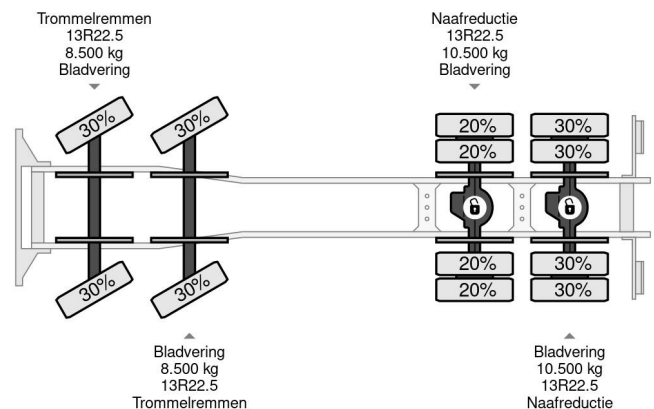
Scania P360 8X4 - EURO 5 + PALFINGER PK22002-EH + R...
