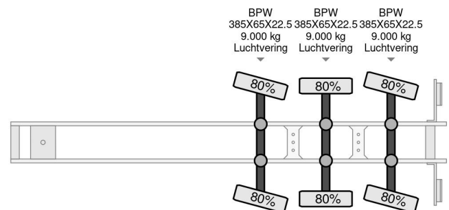
VAN ECK Carrier Maxima 1300
