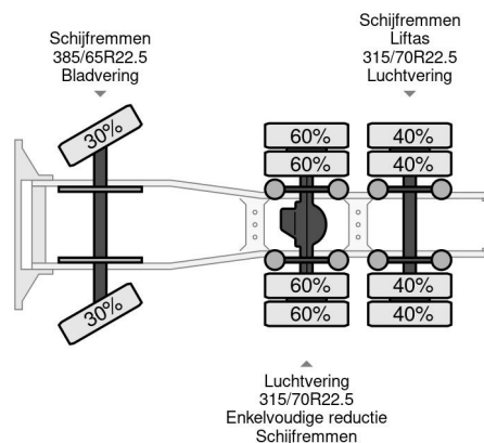
MAN TGX 28.500 6X2 EURO 6 RETARDER DOUBLE AIR
