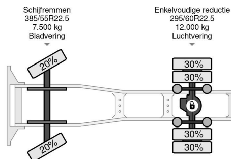
Mercedes-Benz Actros 1842 4X2 - EURO 6 + FULL SPOILER...
