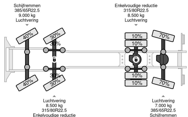
Scania G490 8X4-4 - EURO 6 + MEILLER RK 20 67 HOOK + ...
