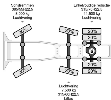
Volvo FH 500 6X2 EURO 5
