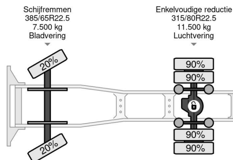
Scania R490 4X2 EURO 6 + ADR RETARDER
